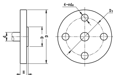
固定法兰 Fixed flange
